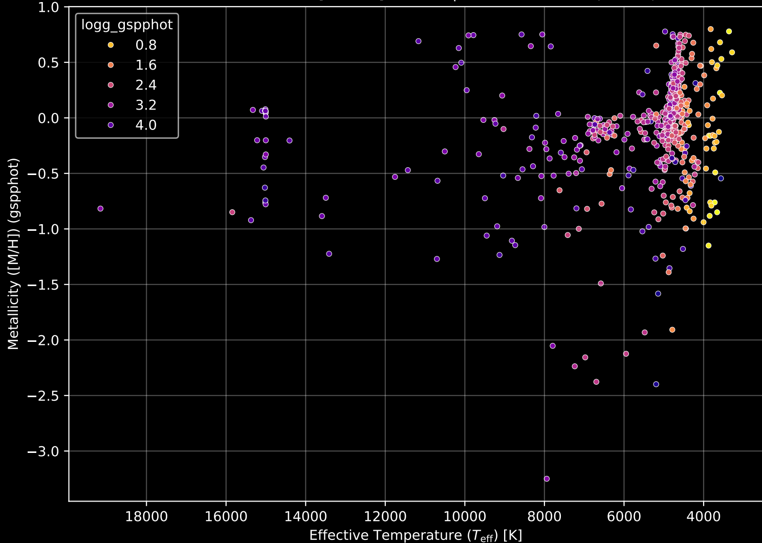
APOGEE DR17 Field: [060+00] Stellar Population Parameters (n= 563)
